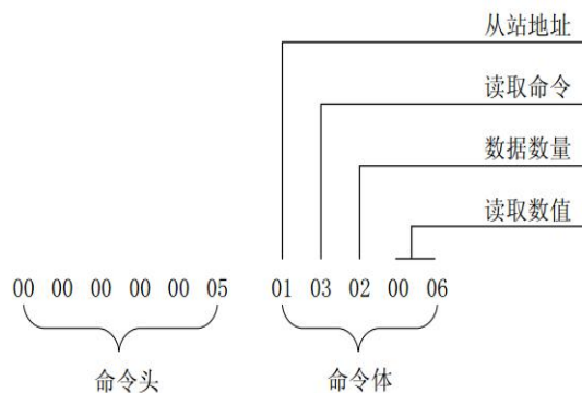
图 4.2 Modbus/TCP 响应帧结构
