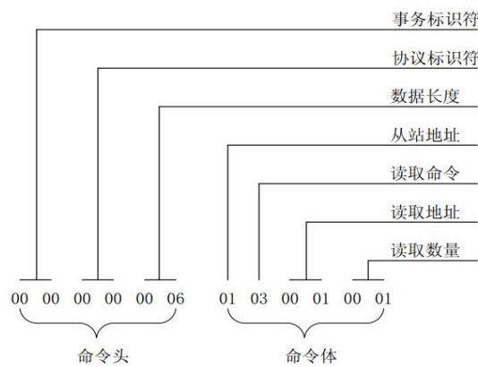
图 4.1 Modbus/TCP 请求命令结构
