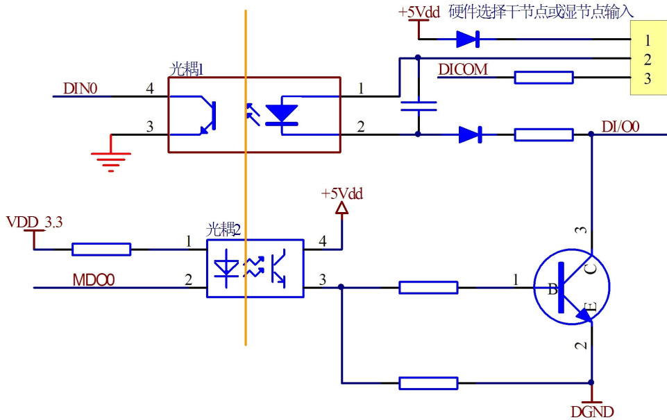
图 2.6 DI/DO 兼容设计端子连接示意图
