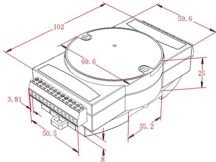
图 1.6 机械尺寸示意图
